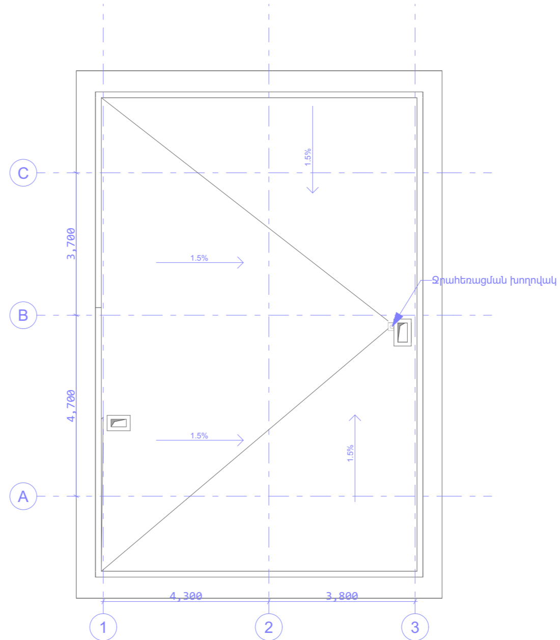
ՏԱՆԻՔԻ ՀԱՏԱԿԱԳԻԾ
