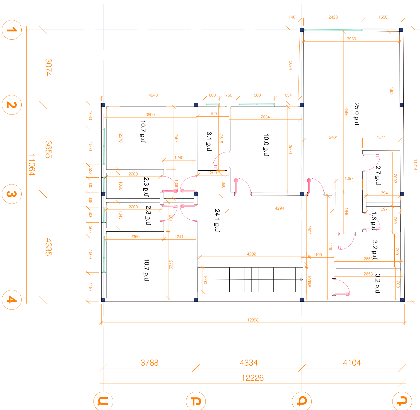
ԵՐԿՐՈՂՂ ՀԱՐԿԻ ՀԱՏԱԿԱԳԻՆ 1:100
