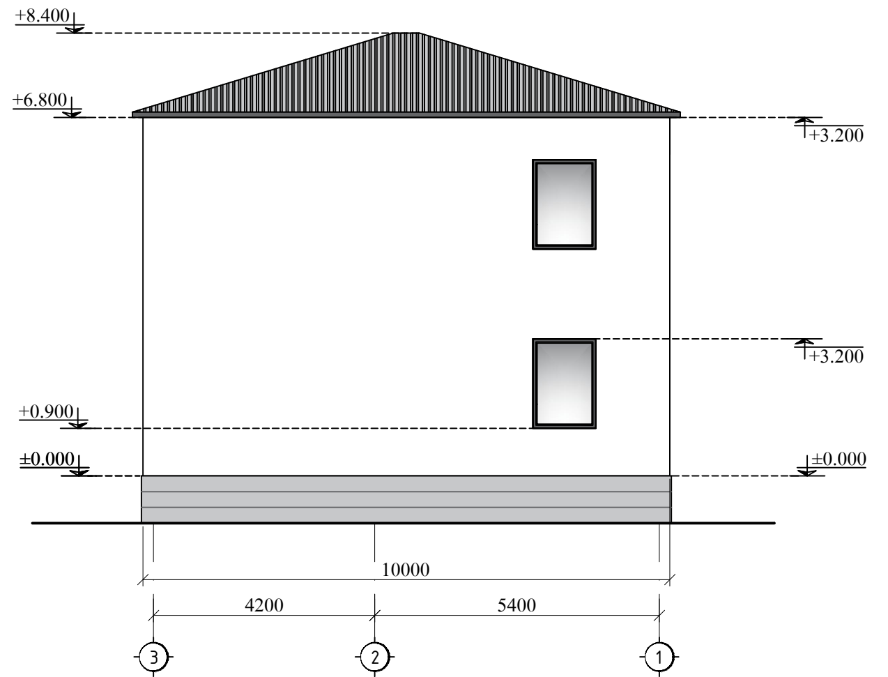
Ճակատ 3-1' առանցքերով Մ 1:100
