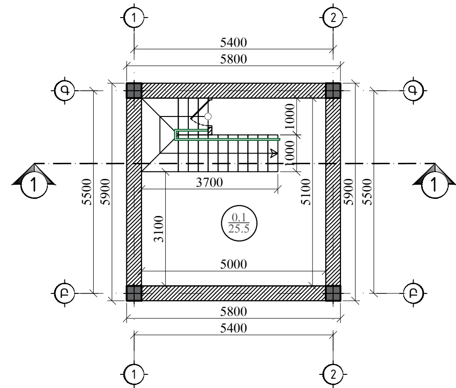
Նկուղային հարկի հատակագիծ - 2.550 նիշում Մ 1:200
