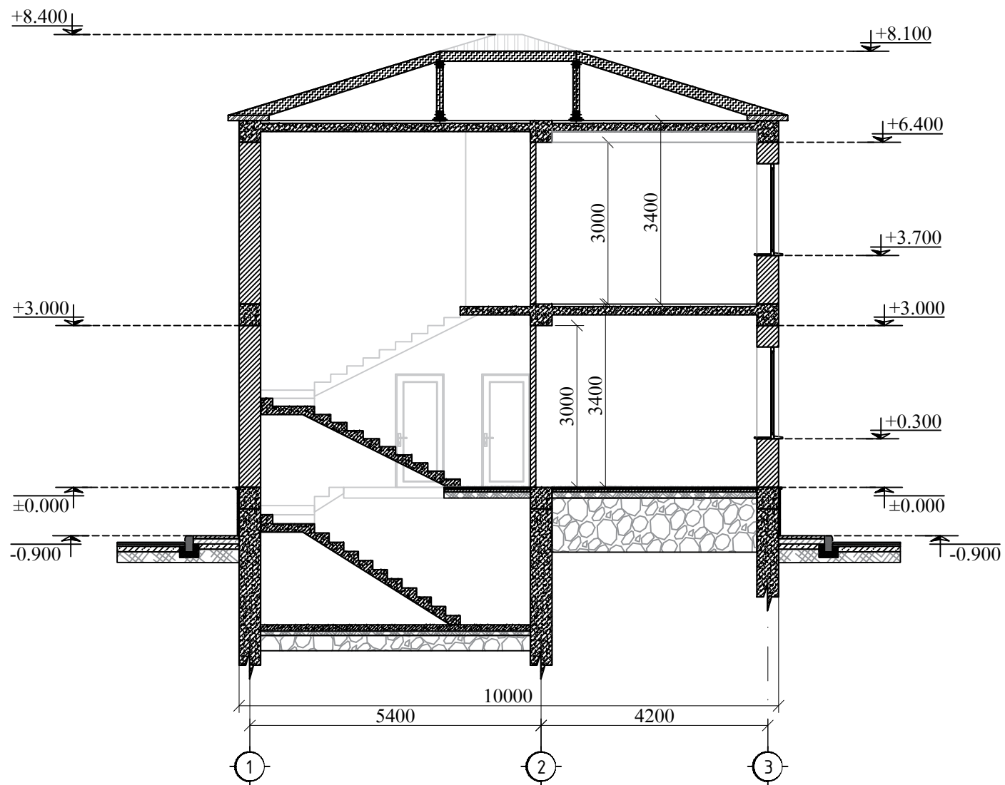
Կտրվածք 3-1 առանցքերով Մ 1:100
