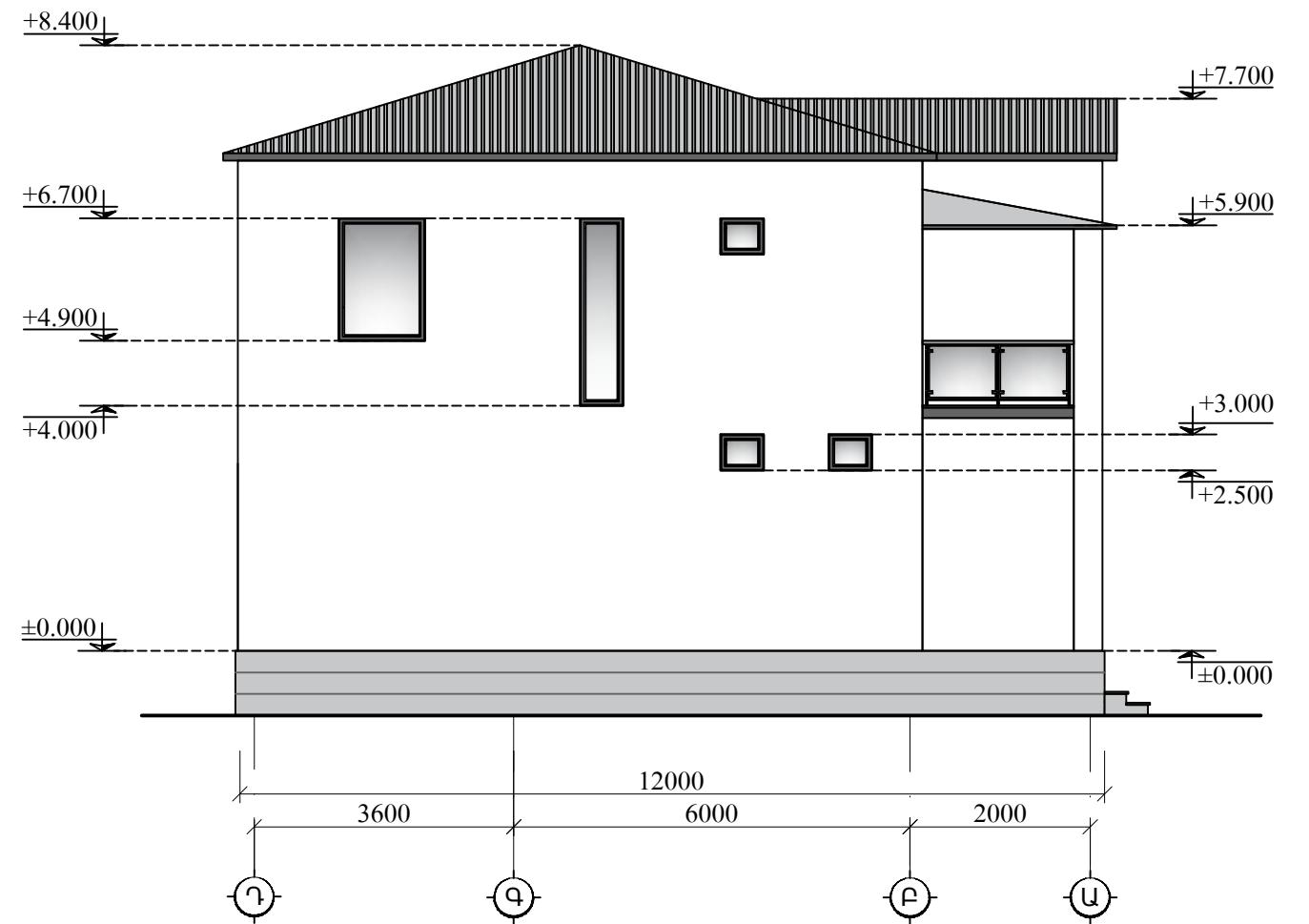
Ճակատ Դ-Ա առանցքներով Մ 1:100
