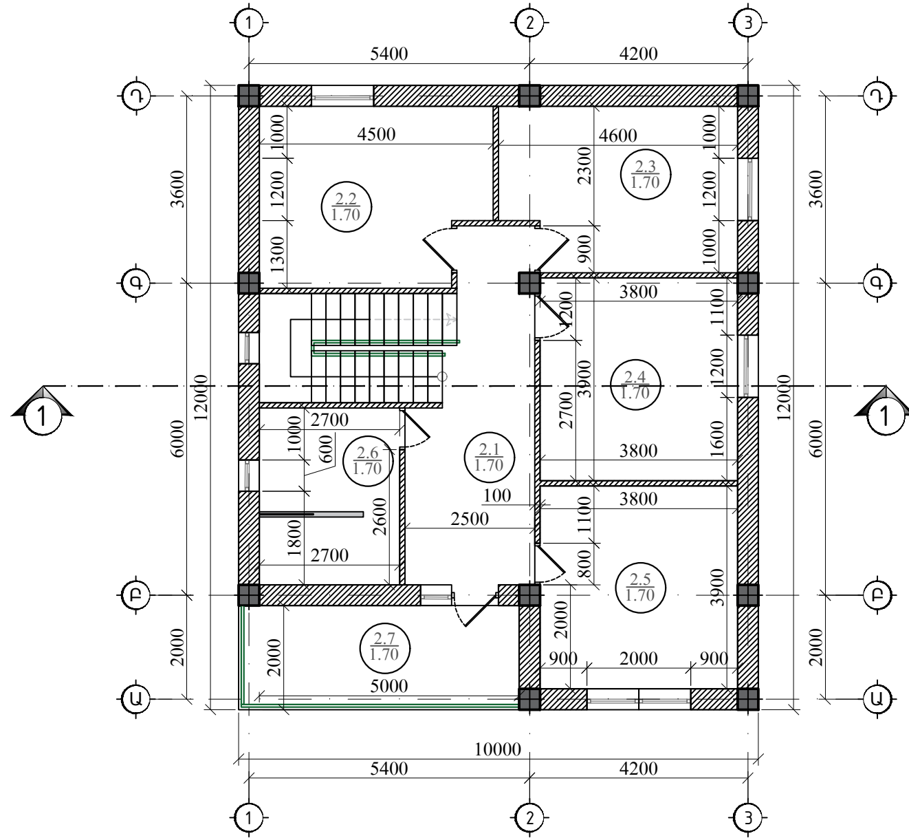
Երկրորդ հարկի հատակագիծ +3.400 նիշում Մ 1:100
