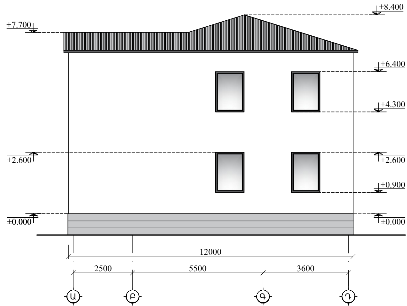
Ճակատ Ա-Դ առանցքներով Մ 1:100
